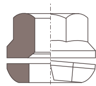
DIN 74361 B/C
