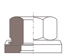
DIN 74361 H
